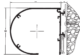
COFFRE ROND LAQUÉ EN ALU EXTRUDÉ
