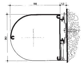
COFFRE SEMI-ROND ALU EXTRUDE AVEC JOUES
